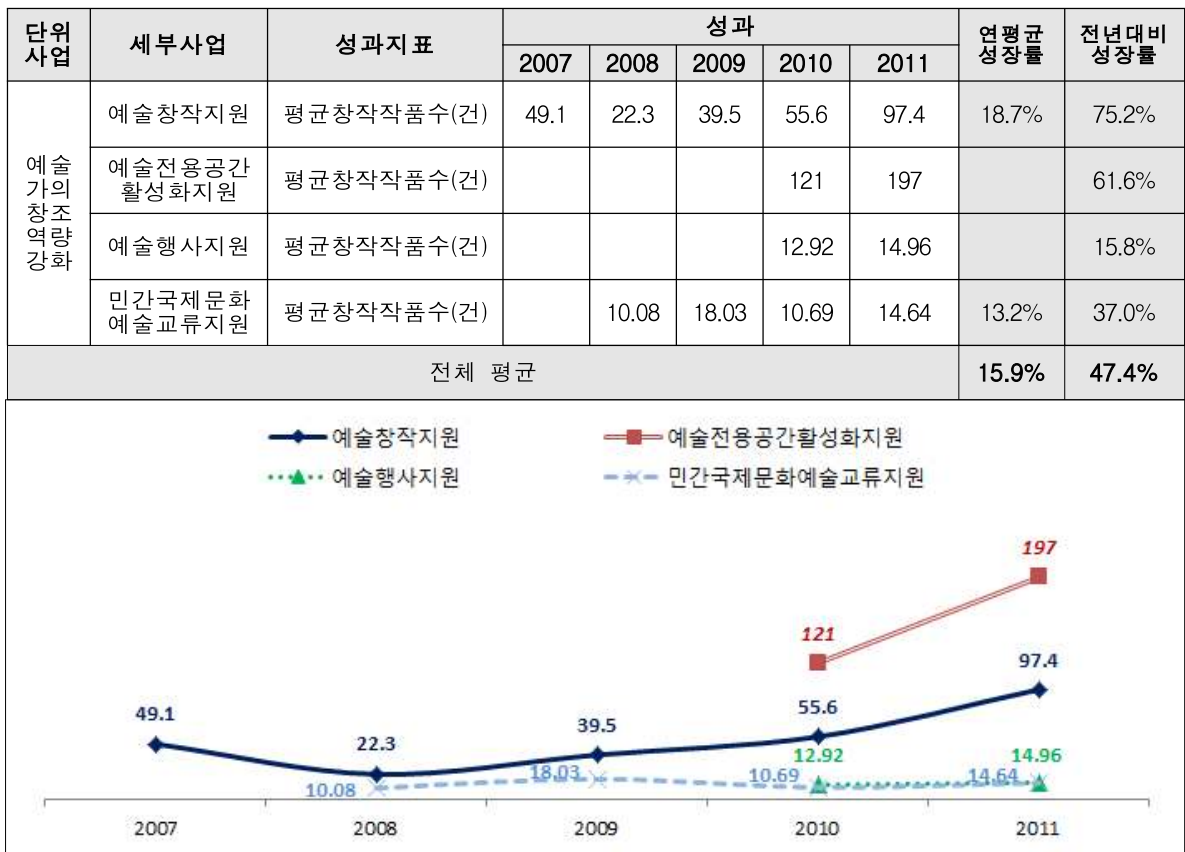
[‘예술가의창조역량강화’의 세부사업별·연도별 평균창작작품수]
